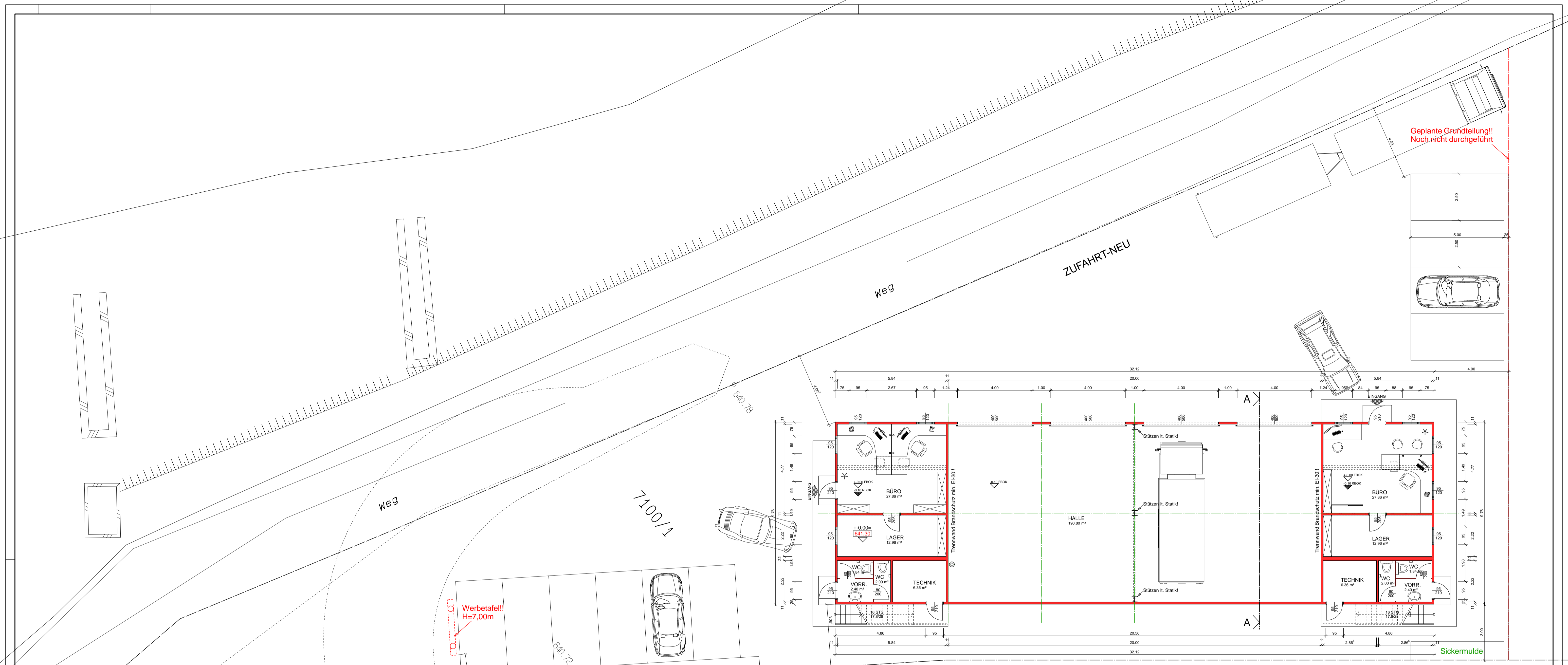
GRUNDRISS ERDGESCHOSS
