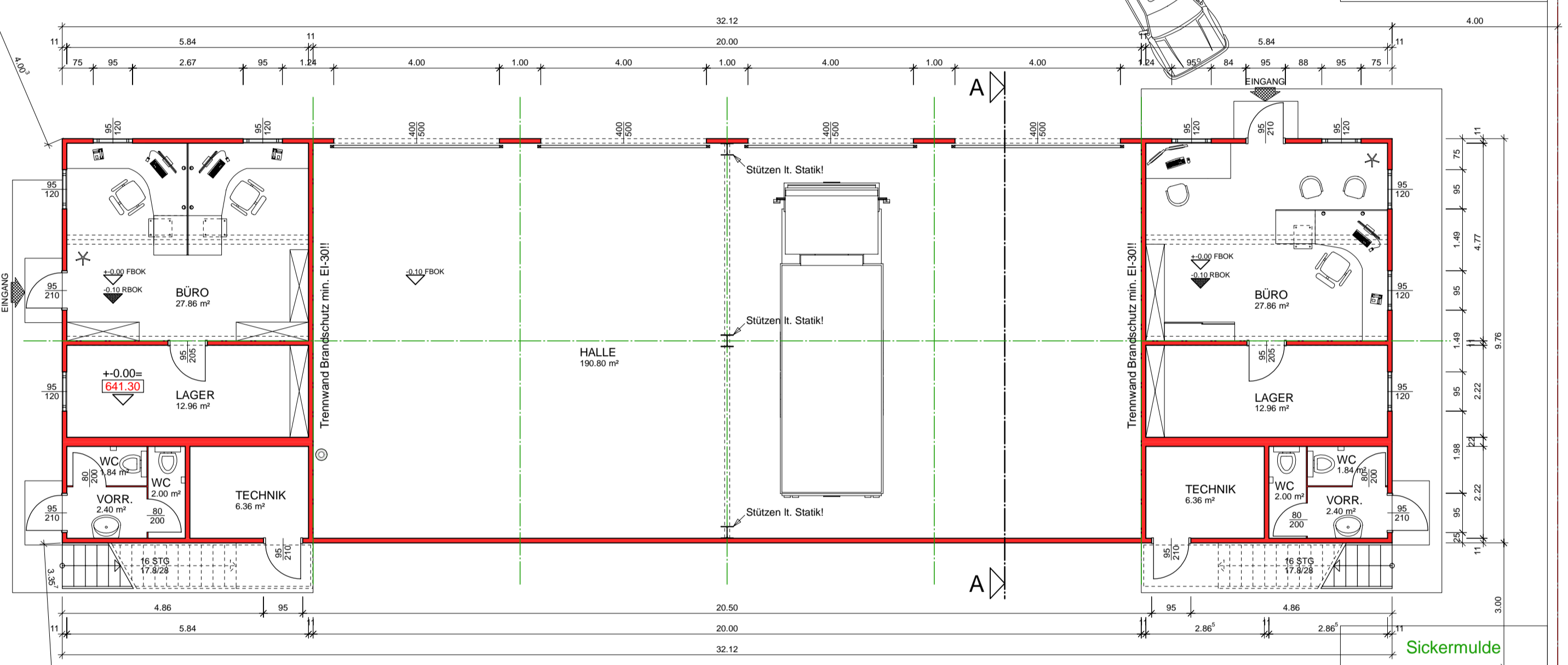
GRUNDRISS ERDGESCHOSS
